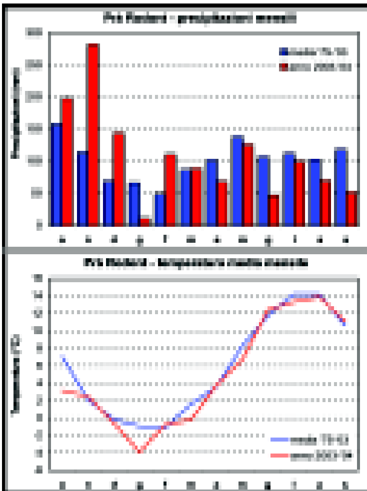
Figura 4. Andamento di precipitazioni e temperature presso la stazione meteorologica di Prà Rodont. I dati dell'anno idrologico 2003-2004 sono messi a confronto con i valori medi del periodo 1975-2003
