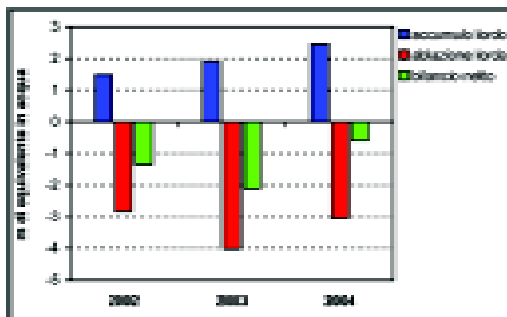
Figura 5. Riassunto dei tre anni di bilancio di massa sul Ghiacciaio d'Agola
